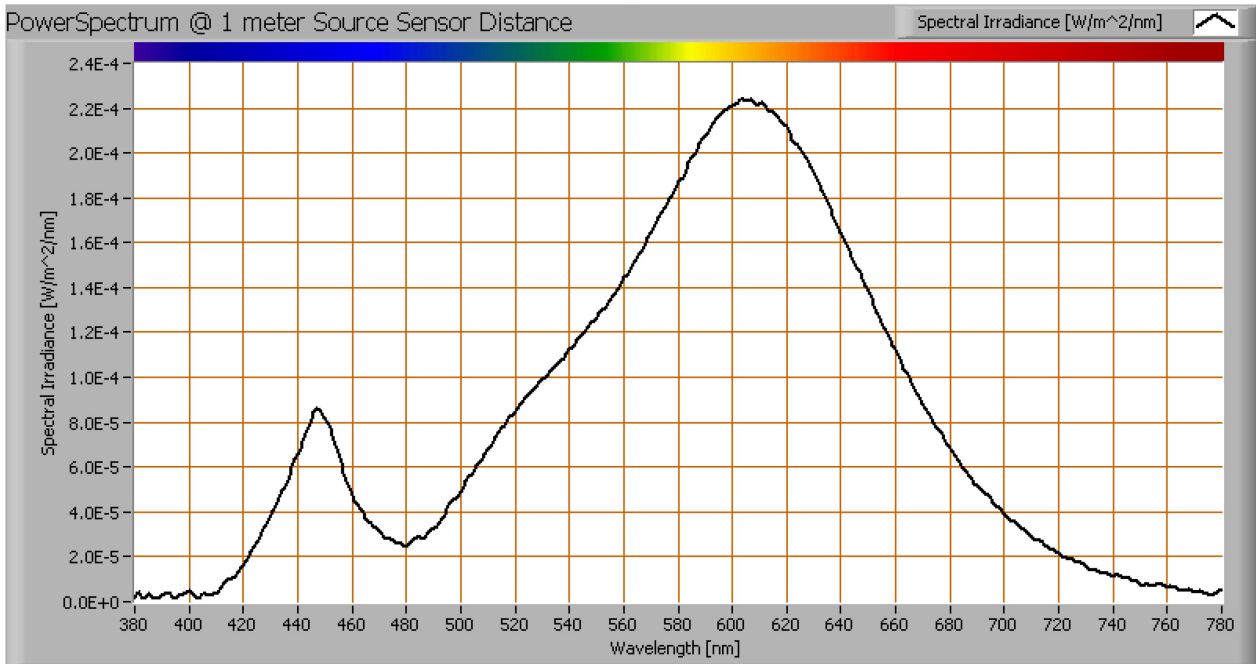
Het kleurspectrum van het licht van deze lamp. Energieniveaus geldig op 1 m afstand.
